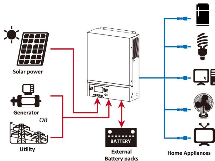
Figura 1 Esquema híbrido
