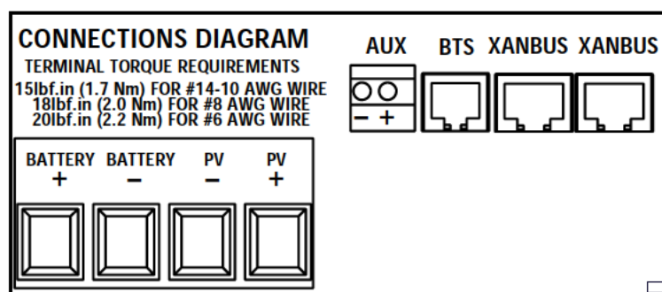
Figura 2-7 Terminales de conexiones de CC
