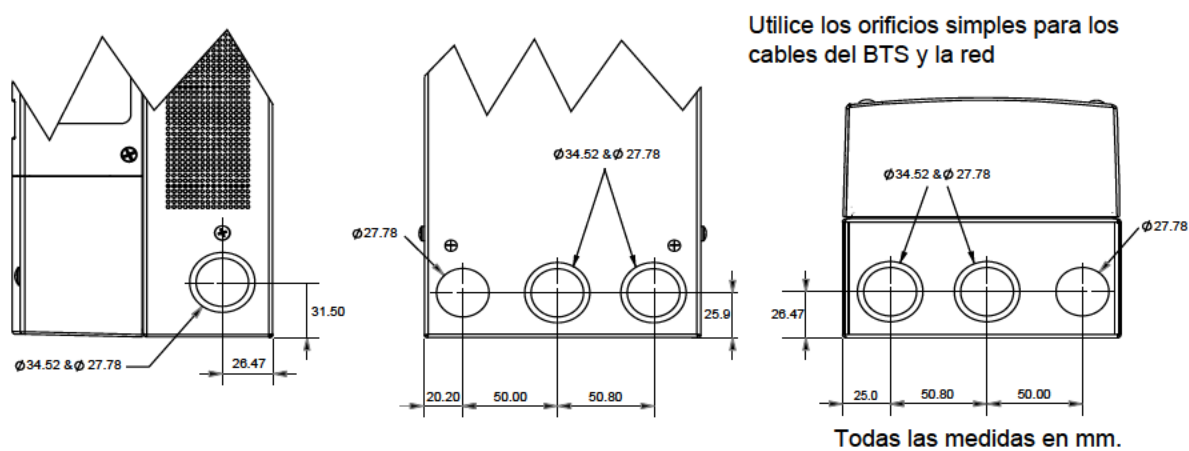
Figura 2-4 Dimensiones de los orificios prehorados
